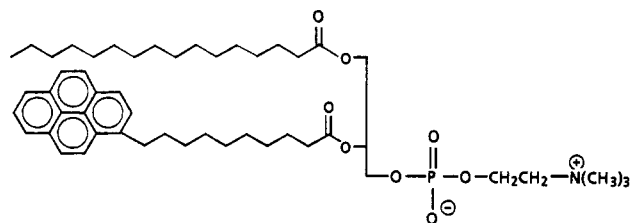
17 PPDP
