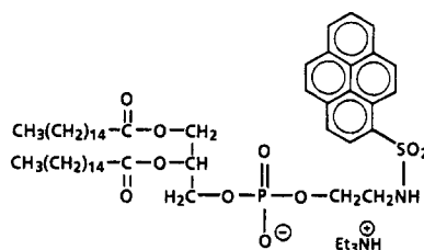
PyDPPE
